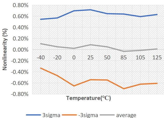
图 5: 非线性度 Vs 环境温度
