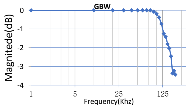
图 8: -3db 带宽
