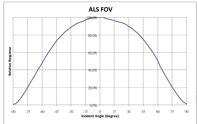
ALS FOV
