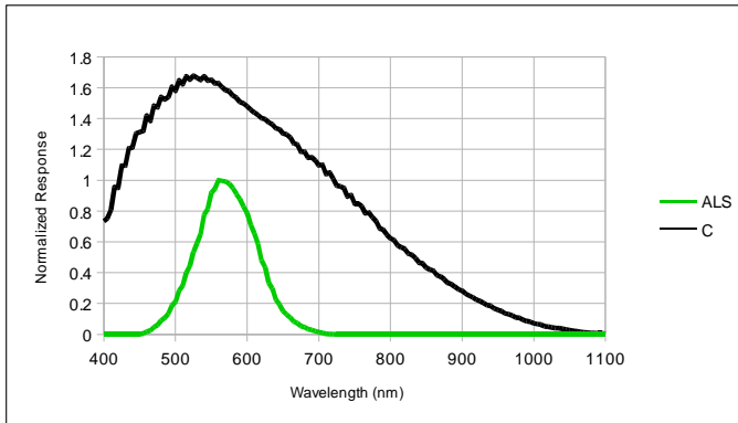
ALS Spectrum
