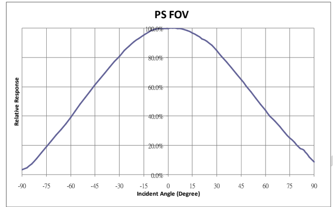
PS FOV
