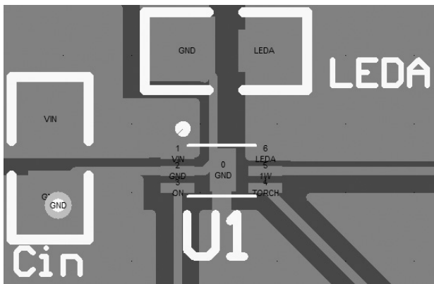
图 6. UDFN-1.5x2-6L 的 PCB 布线图
