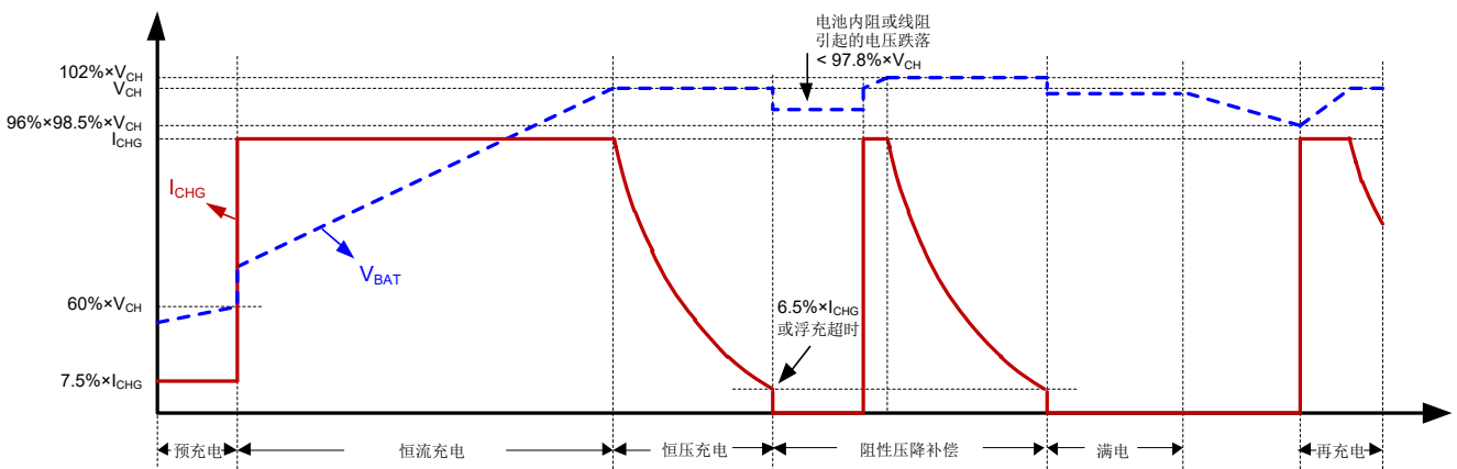
图 5. SGM40560A 充电周期示意图 (阻性压降大于 2.2\% \times V_{CH} )
