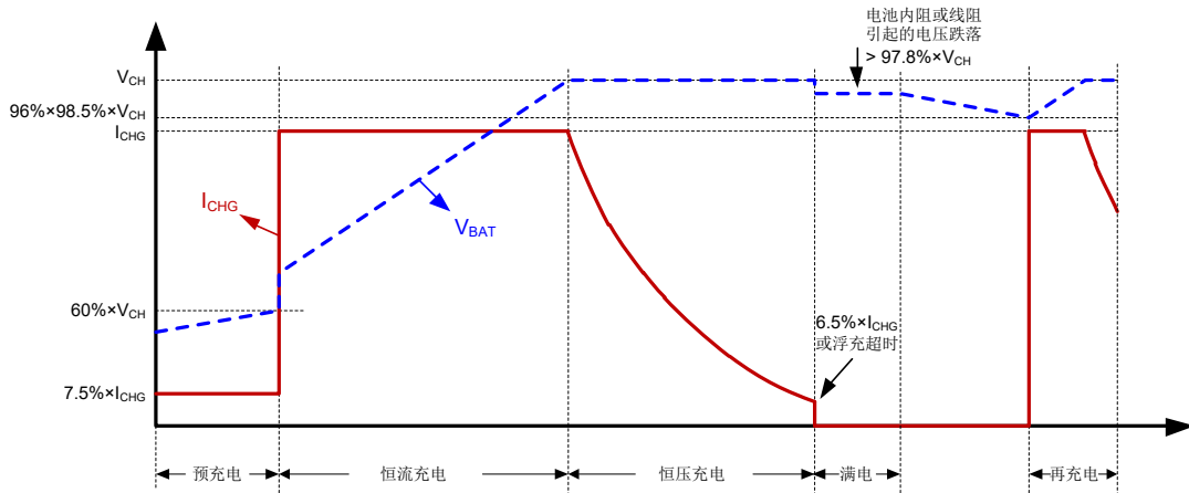
图 4. SGM40560A 充电周期示意图 (阻性压降小于 2.2\% \times V_{CH} )
