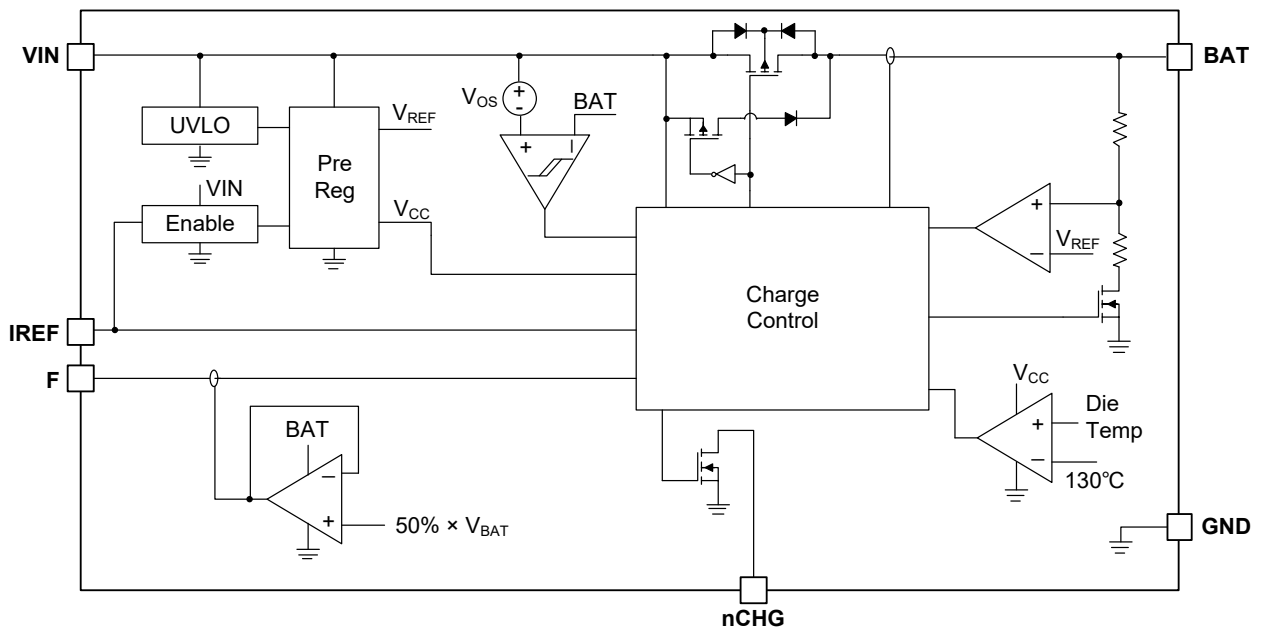
图 2. SGM40560A 内部原理示意
