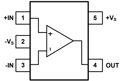
SOT-23-5/SC70-5
