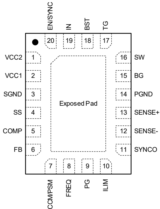
TQFN-3x4-20L
