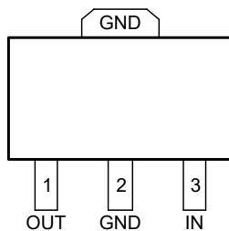
SOT-89-3
