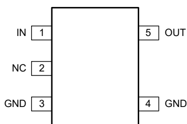
SOT-23-5
