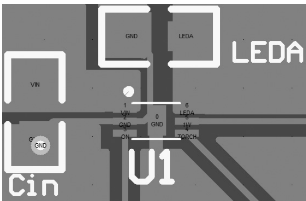
图 6. UDFN-1.5x2-6L 的 PCB 布线图
