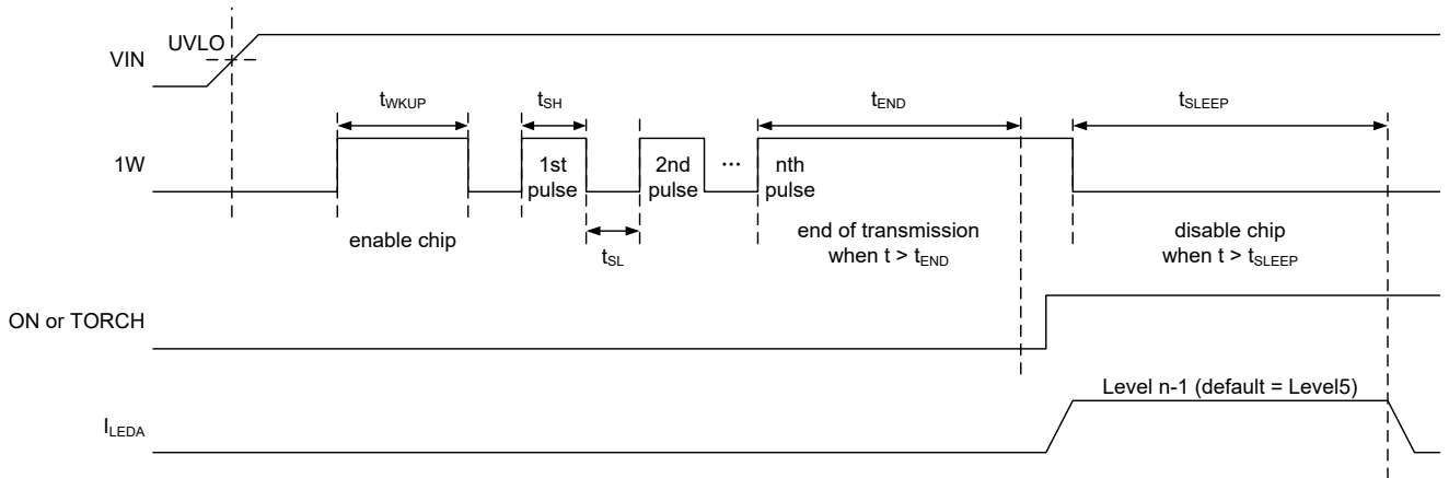
图 3. 可编程的 1W 时序图
