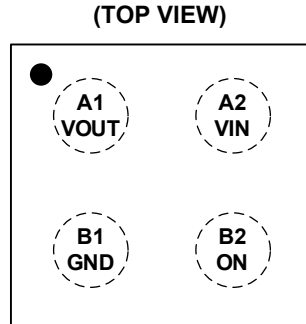
WLCSP-0.9×0.9-4B-A
