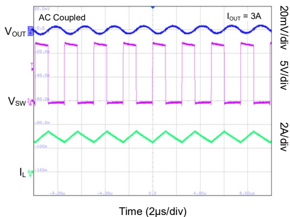
SGM61330A CCM Mode
