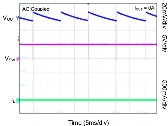
SGM61330A PFM Mode
