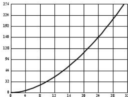
图 6 伽玛补偿修正曲线 (32 级)
