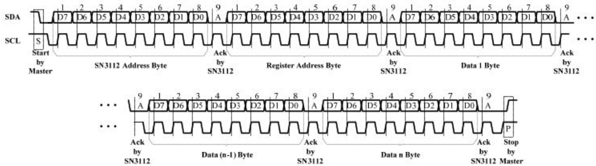
图5 地址自加方式写入 SN3112-12
