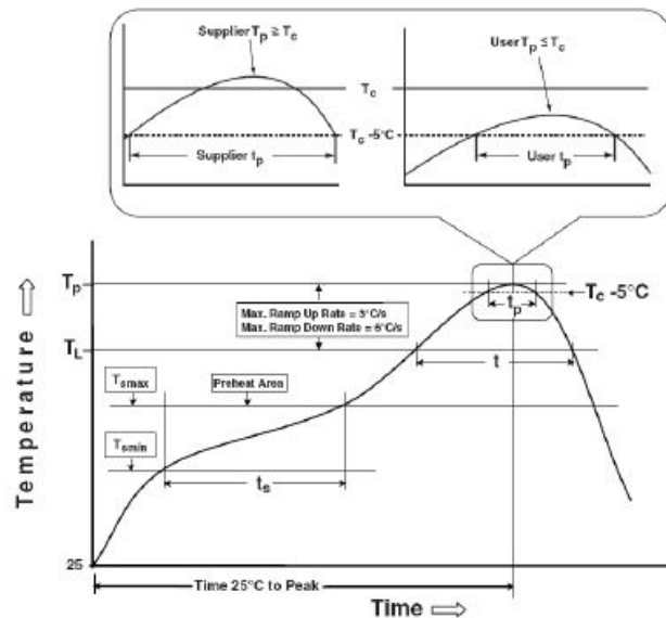
图8 回流焊接温度曲线
