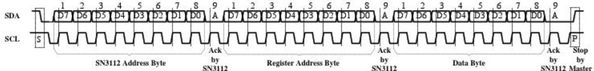
图4 典型方式写入 SN3112-12
