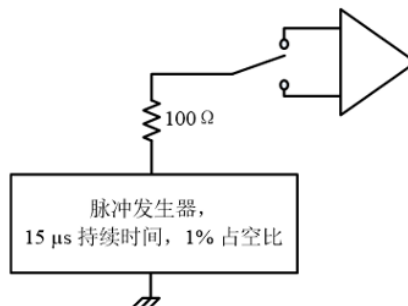
图 9 过压保护
