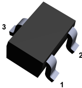
SOT323-3L (Jedec SC-70)
