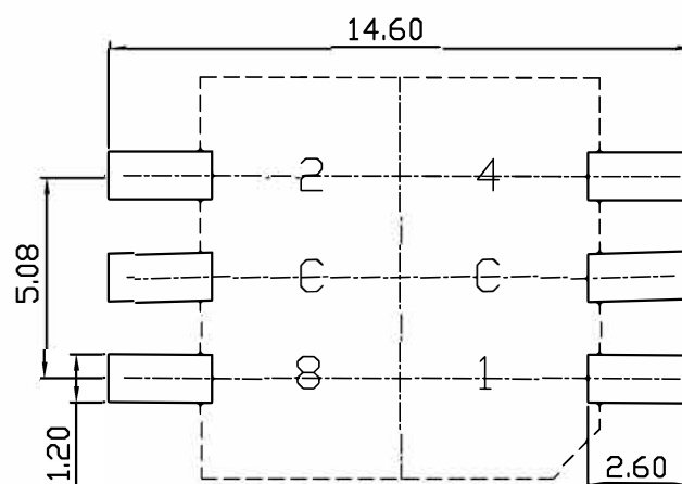
P.C.B DIMENSION
