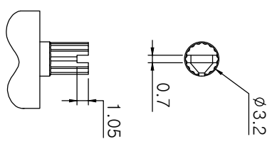
ACTUATOR
