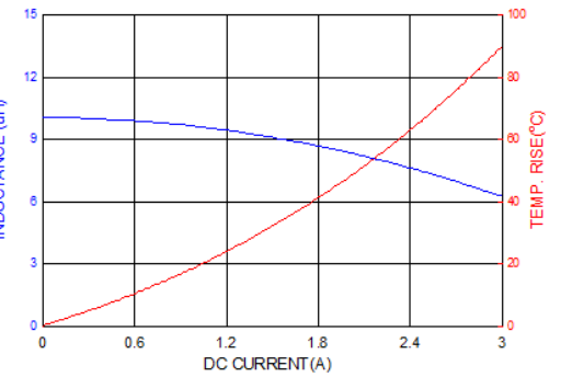
PICQ0415HP100MF
