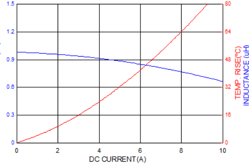
PICQ0415HP1R0MF
