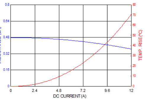
PICQ0415HPR47MF
