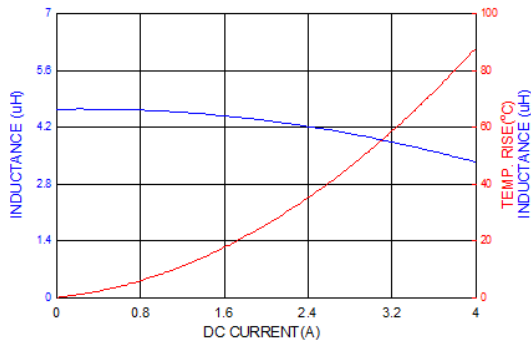
PICQ0415HP4R7MF
