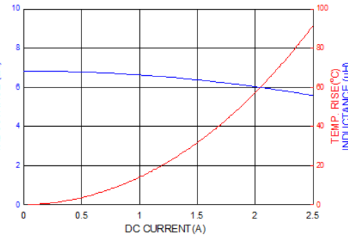
PICQ0415HP6R8MF
