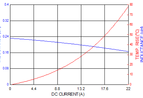
PICQ0415HPR22MF
