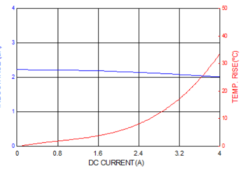
PICQ0415HP2R2MF
