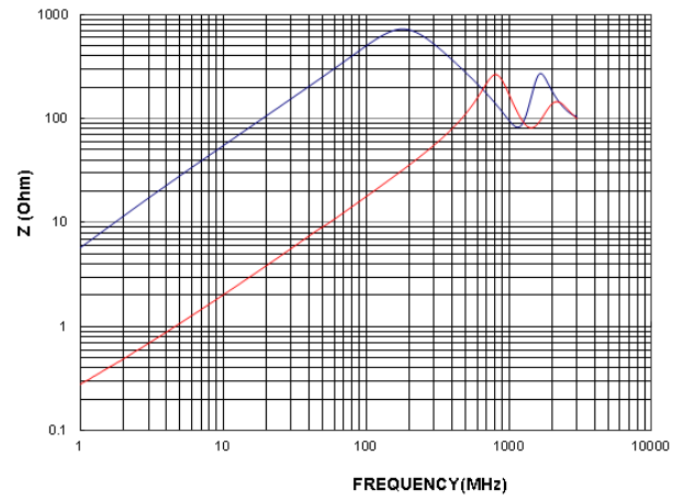
WCM5025F2SF-501T40
