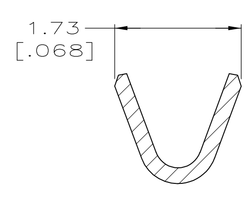
SECTION A-A SCALE 20:1
