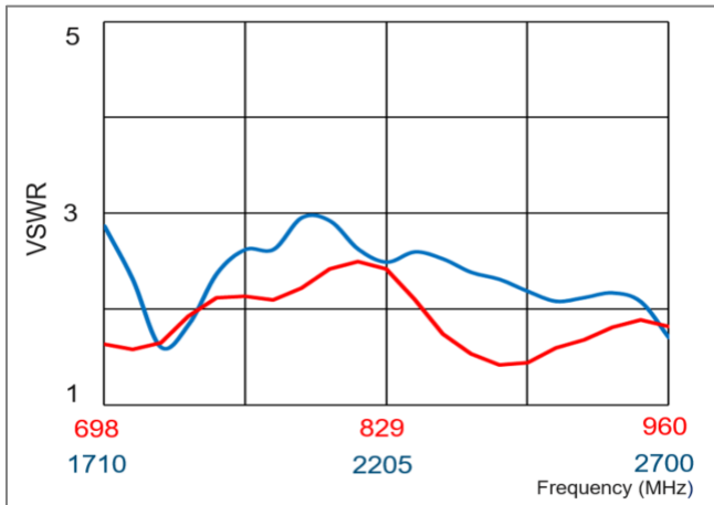
VSWR
