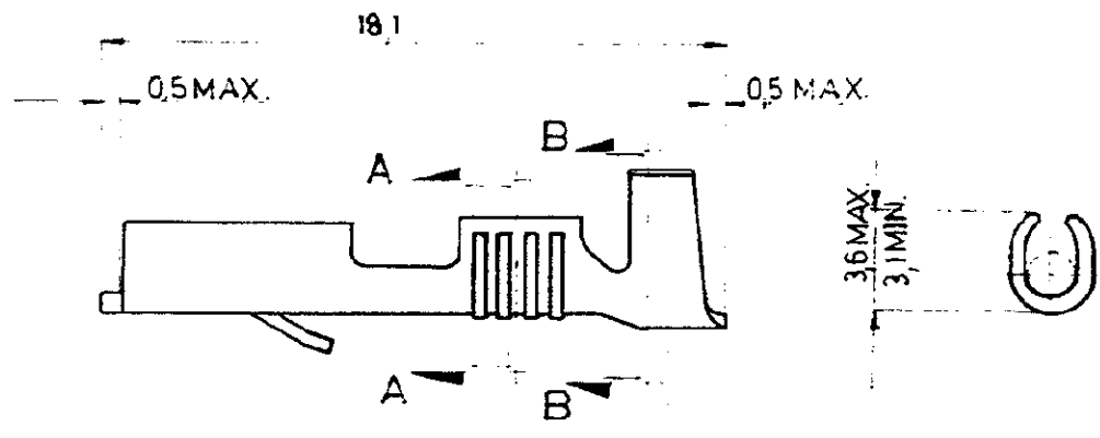
SECCION-A-A
