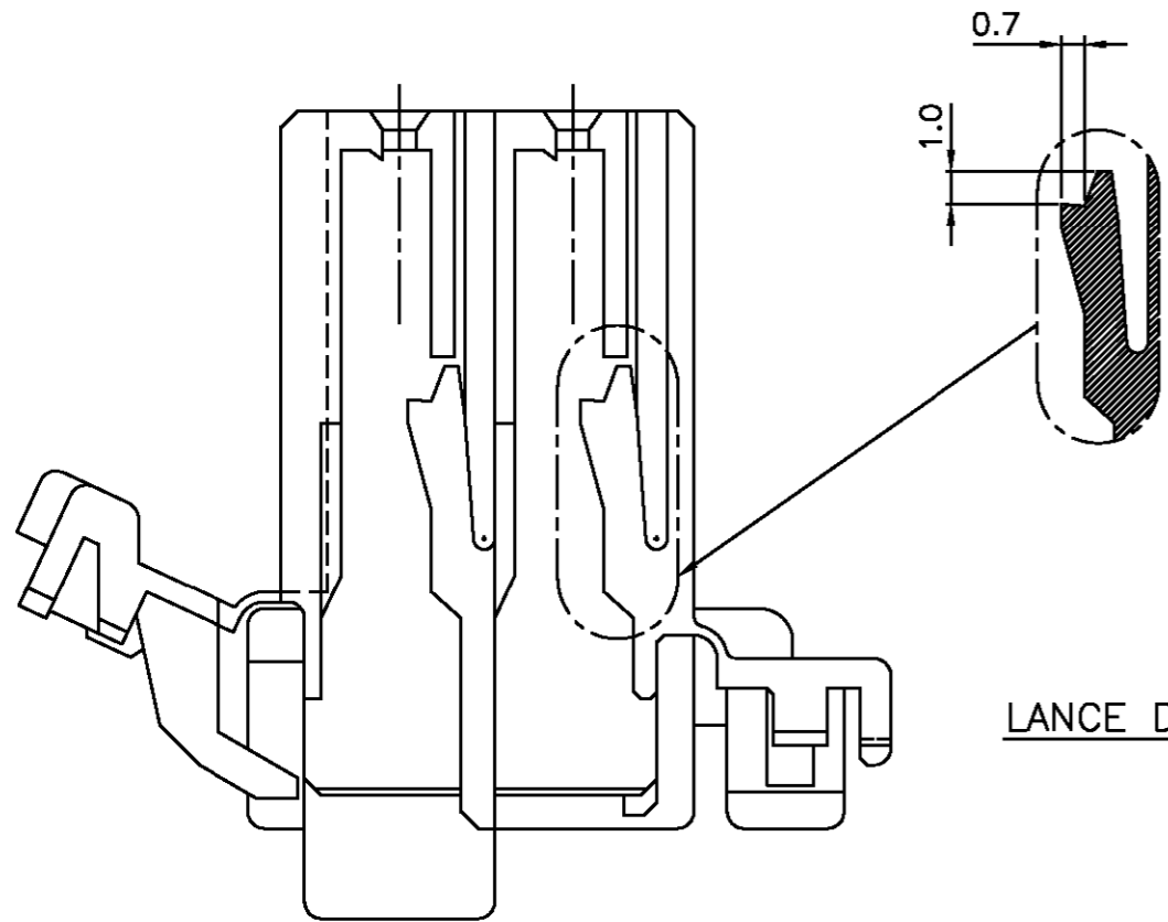
SECTION A-A
