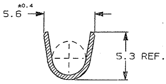
SEZIONE B-B (SECTION B-B)
