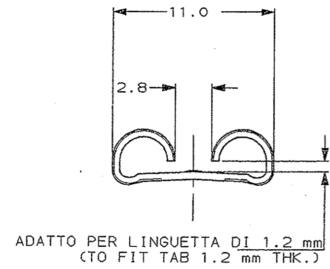
SEZIONE A-A (SECTION A-A)
