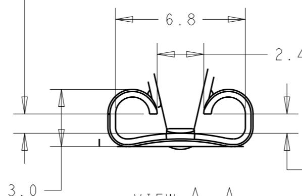
VIEW A-A
