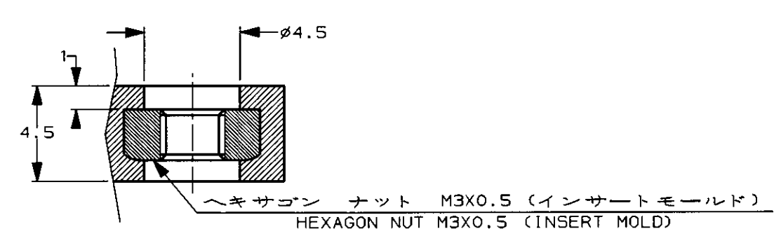
SECT A-A
