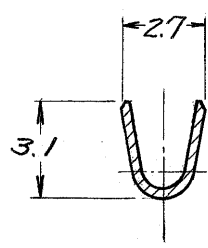
断面 B-B
