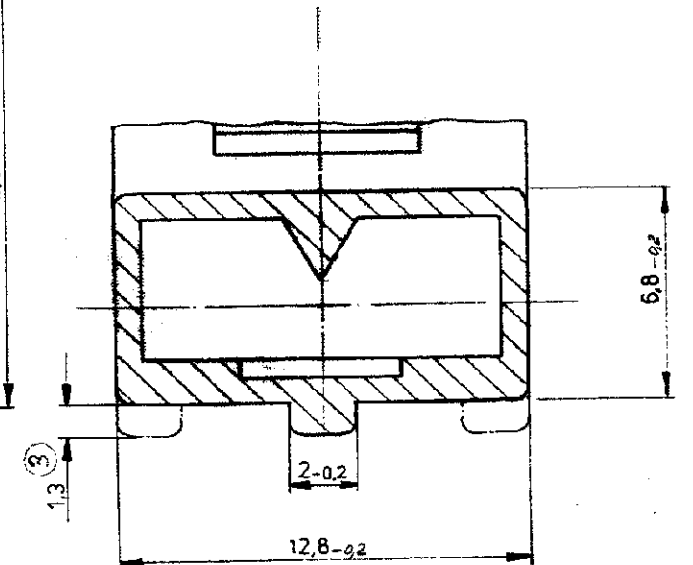
SCHNITT A-A
