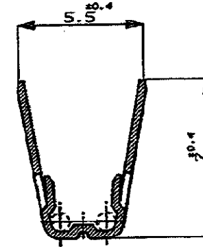
断面 A-A SECT. A-A
