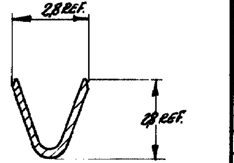
SECCÃO A-A ESC. 8:1
