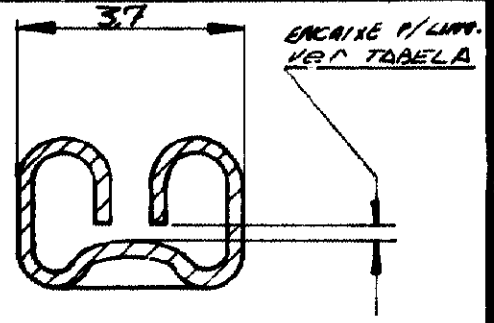
SECCÃO B-B ESC. 8:1
