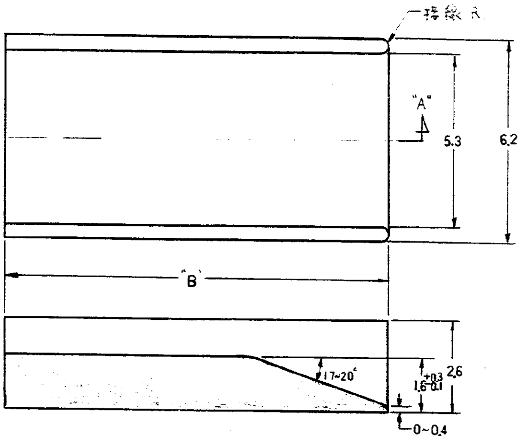
断面 "A-A"
