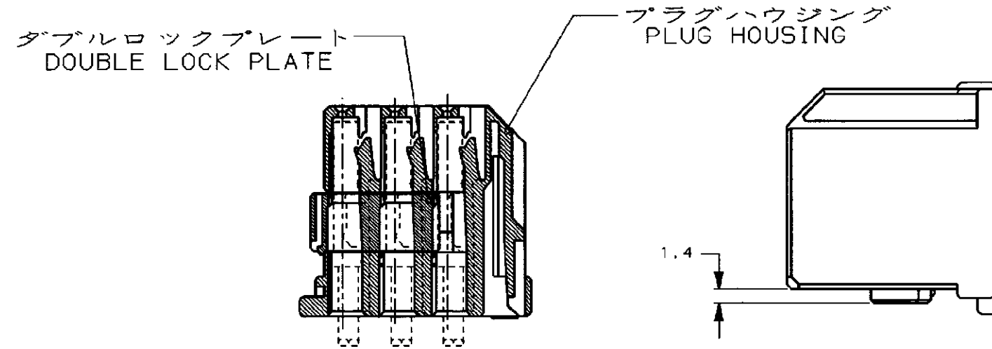
断面 A-A (SECT. A-A)
