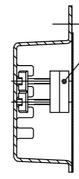
SECTION C-C SCHNITT C-C
