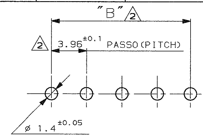
DIMA DI FORATURA SU C.S. (RECOMMENDED P.C.B. HOLE PATTERN)
