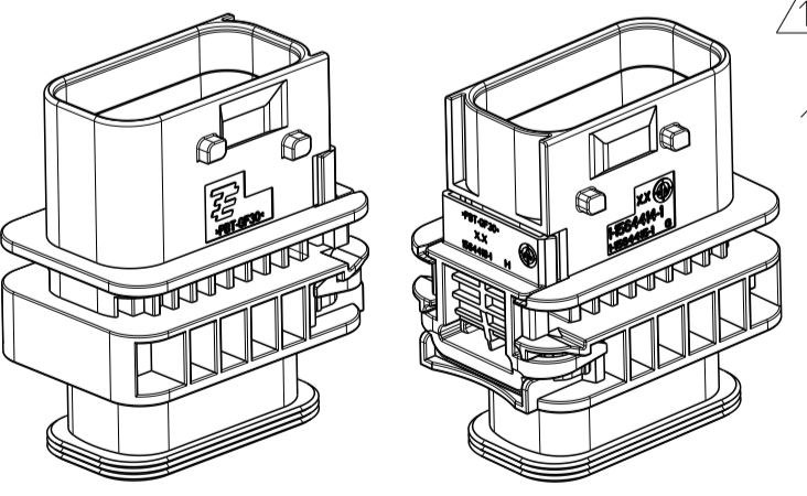
SCALE 1:1 Massstab
