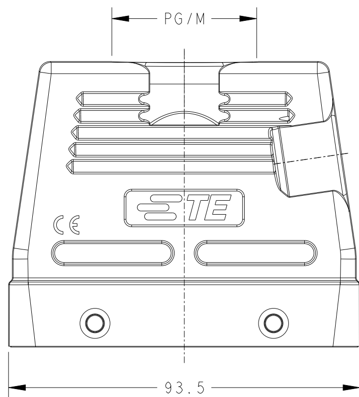
SCALE 1:2
