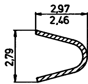
SCHNITT E-F
