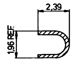
SCHNITT C-D
