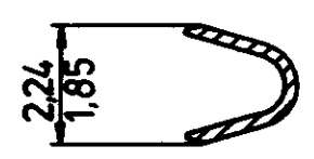
SCHNITT A-B
