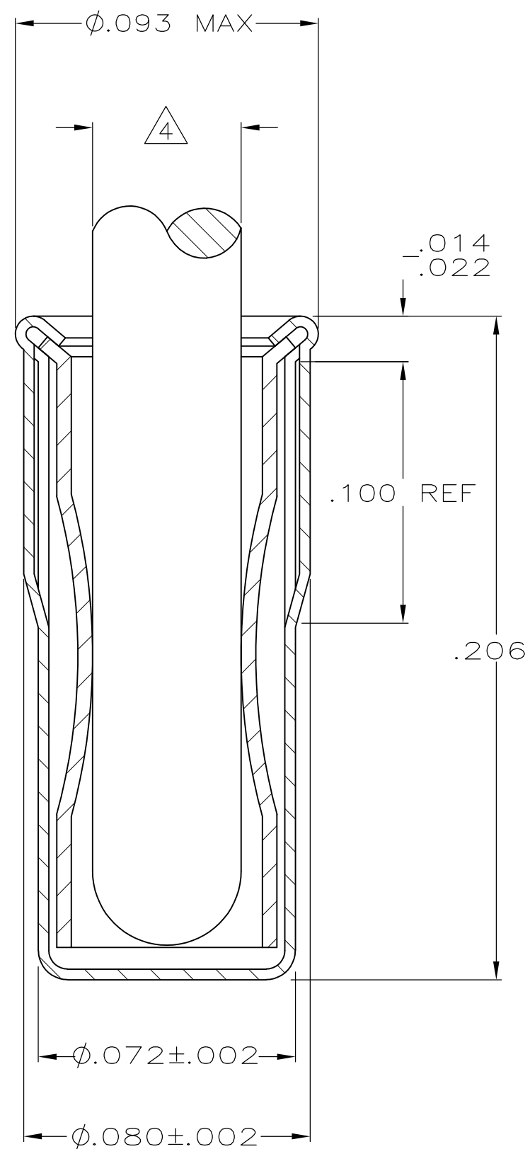
SECTION A-A
