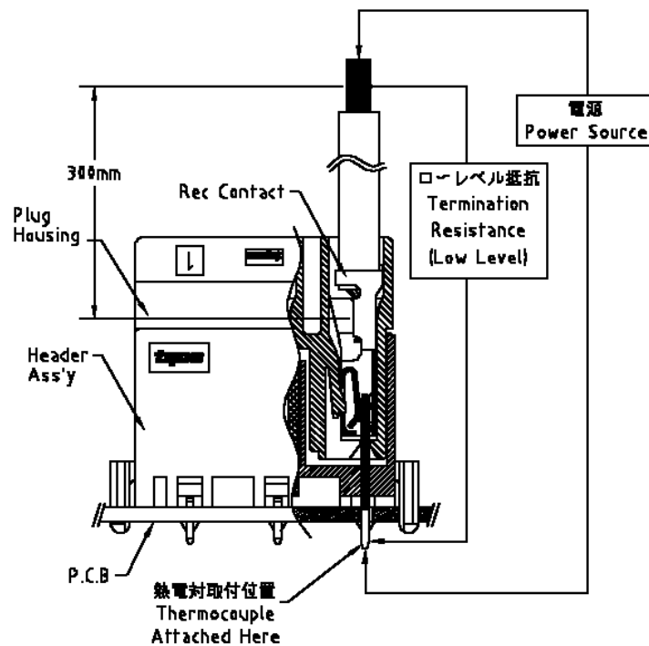
Fig. 8-2 温度上昇
