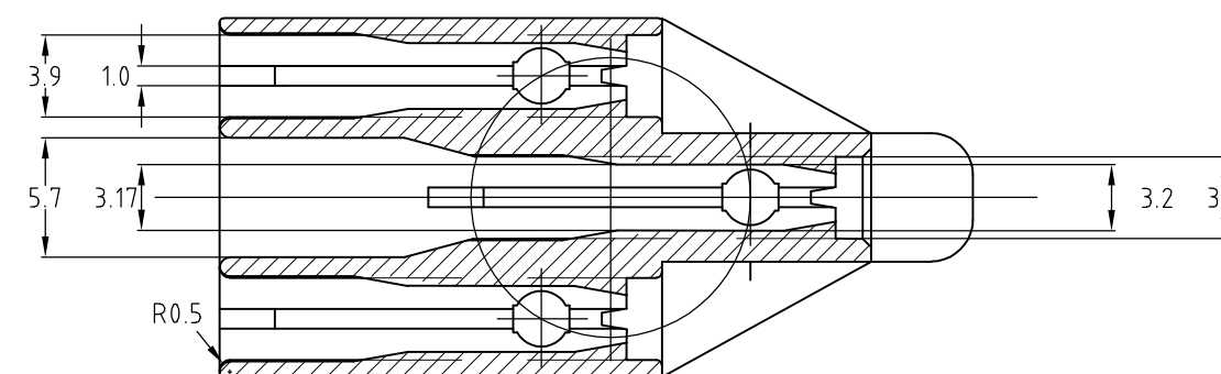
断面 B-B
