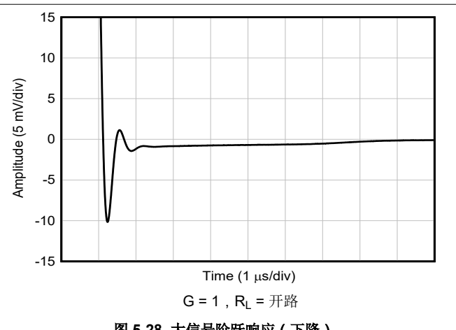
图 5-28. 大信号阶跃响应 (下降)
