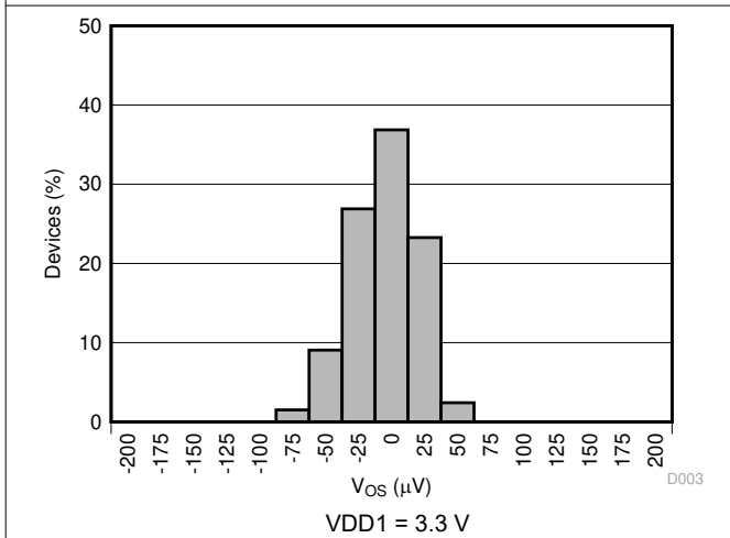
图 6-7. Input Offset Voltage Histogram
