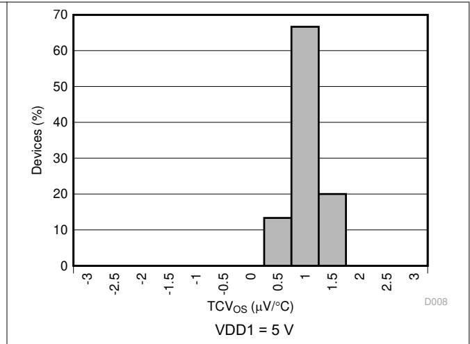
图 6-12. Input Offset Drift Histogram
