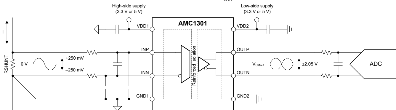
简化原理图
