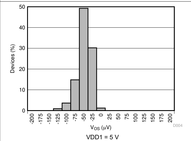
图 6-8. Input Offset Voltage Histogram
