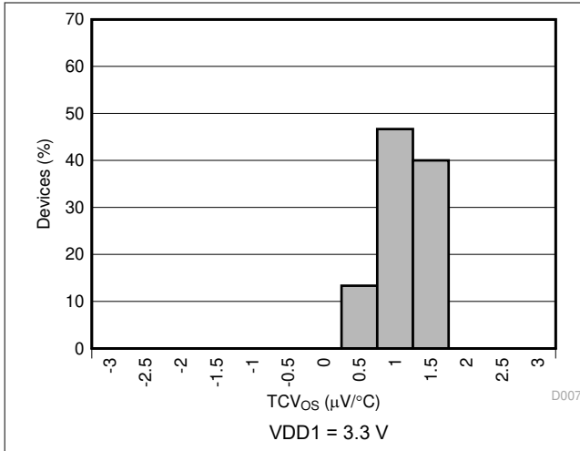
图 6-11. Input Offset Drift Histogram
