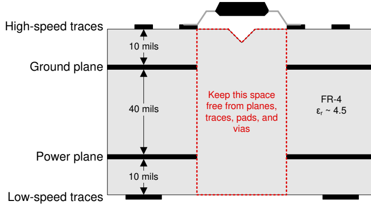
图 11-1. 建议的层堆叠
