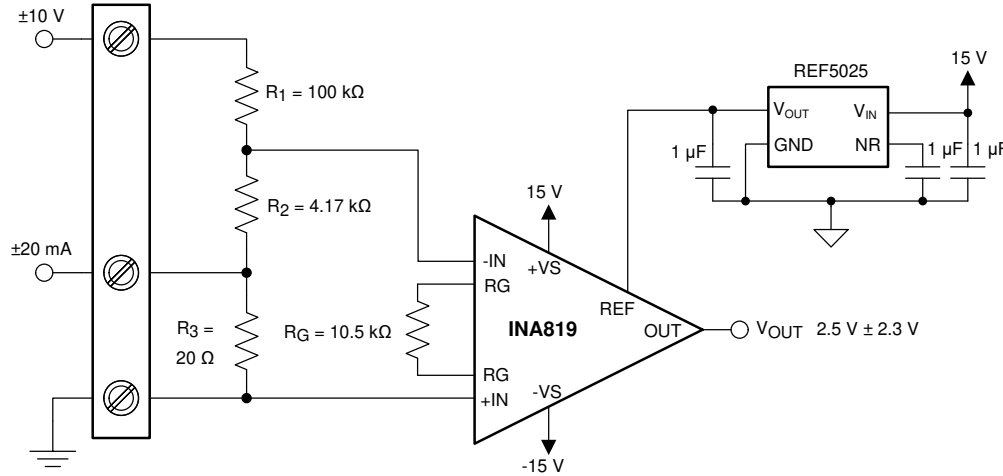
图 9-5. PLC Input (±10 V, 4 mA to 20 mA)
