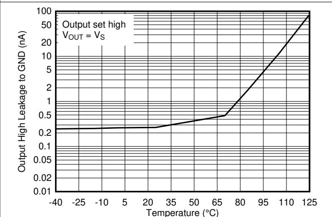
图 6-29. 36V 下输出高电平漏电流与温度之间的关系
