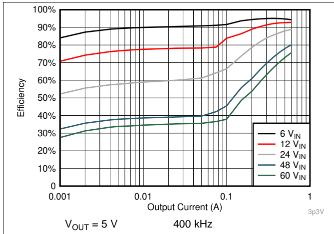
图 22. Efficiency
