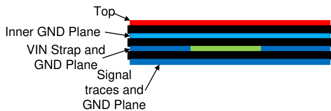
图 54. Example Layout
