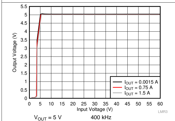
图 26. Line Regulation
