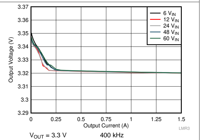
图 25. Load Regulation
