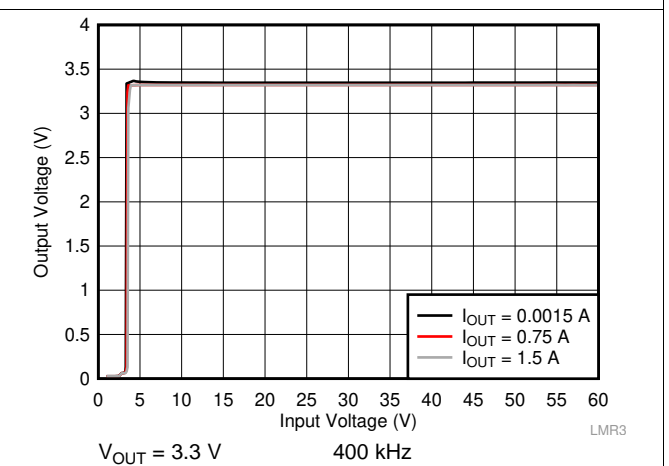
图 27. Line Regulation
