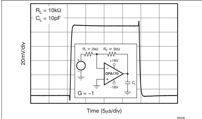
图 29. 小信号阶跃响应 (100mV)
