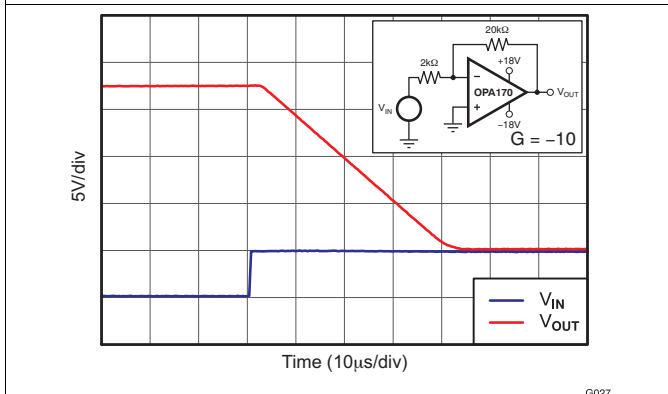
图 27. 负过载恢复
