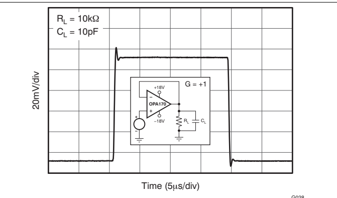
图 28. 小信号阶跃响应 (100mV)
