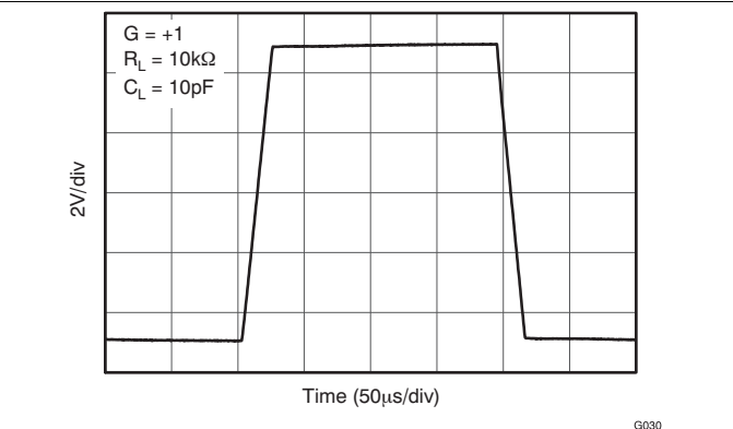
图 30. 大信号阶跃响应
