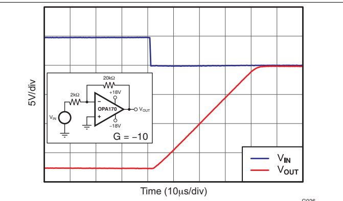
图 26. 正过载恢复
