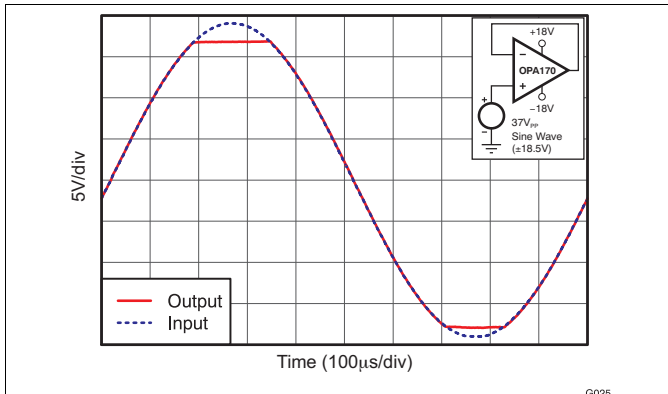
图 25. 无相位反转
