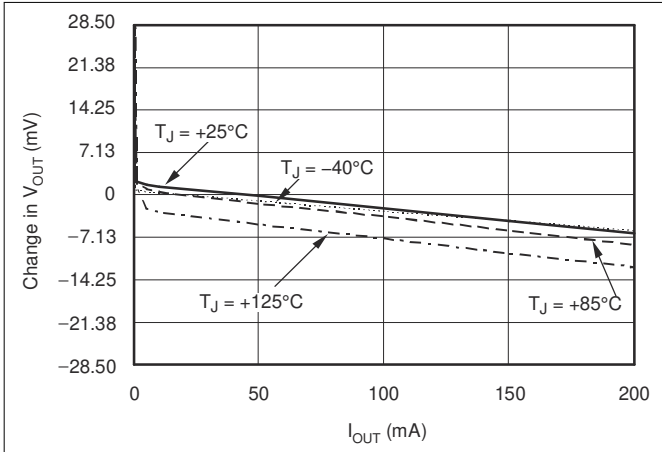
图 6-1. Load Regulation
