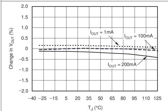
图 6-1. Load Regulation
