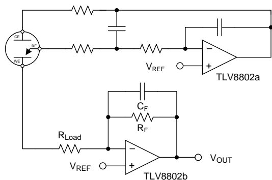
毫微功耗电化学传感器放大器
