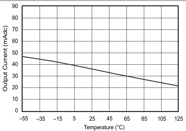
图 6-48. 拉电流限制
