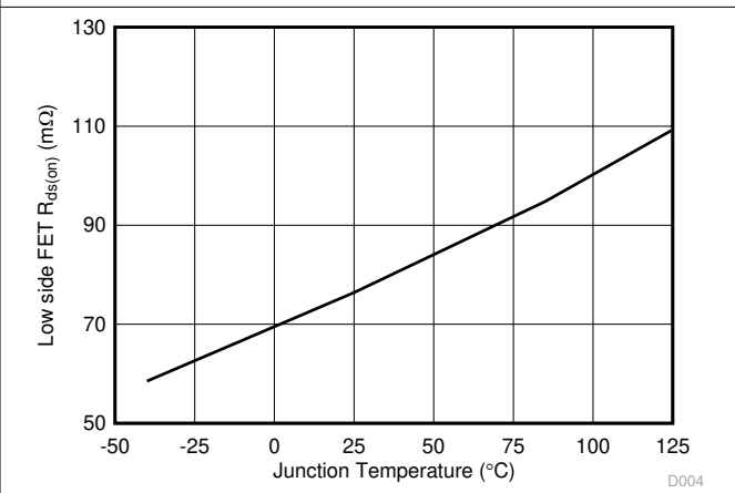
图 6-4. 低侧 FET 导通电阻与结温间的关系
