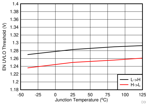
图 6-11. EN UVLO 阈值与结温间的关系
