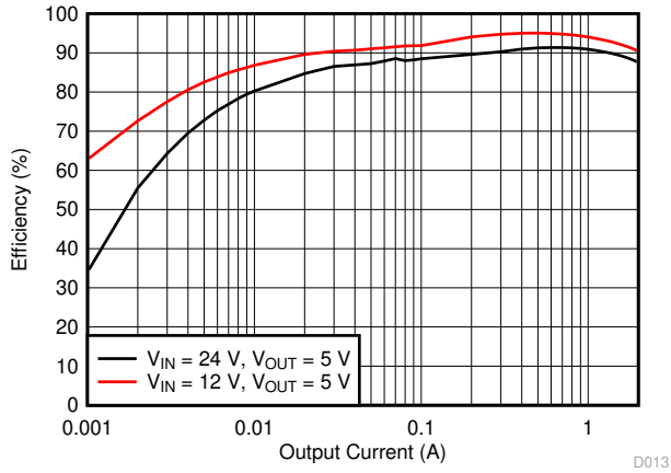
图 8-2. 效率
