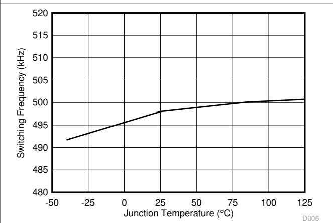
图 6-6. 中央开关频率与结温间的关系
