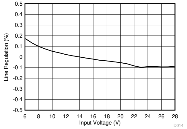
图 8-3. 线路调节
