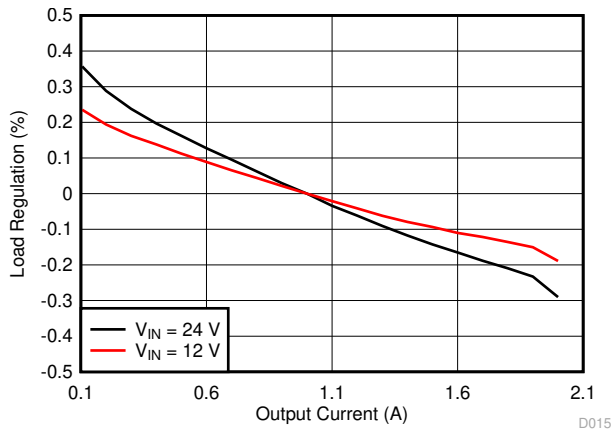
图 8-4. 负载调节
