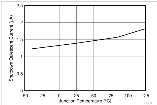
图 6-1. 关断静态电流与结温间的关系
